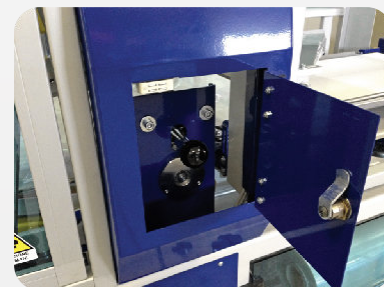
Gruppo controllo traino film Film pulling guard
